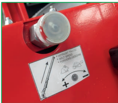
Geschwindigkeitsverstellung des Förderbands
